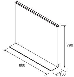
Espejo BECKET 800 horizontal con luz led (9 W - 5700°K) IP 44 estante inferior negro incluido 800 x 790 mm 105600
