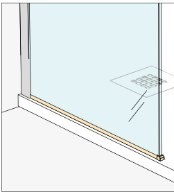
Perfil a suelo para cristal fijo de 8 mm
