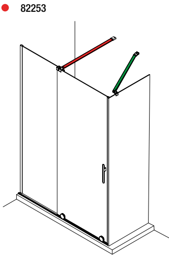
Mampara angular compuesta por un frontal, con tensor frontal y con lateral fijo. (pag 164)
