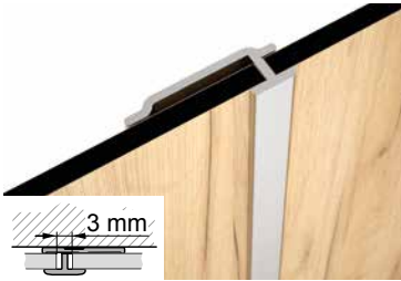
Perfil unión paneles frontales
