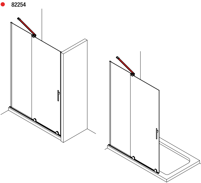
Mampara frontal compuesta por tensor angular (pag 162)
