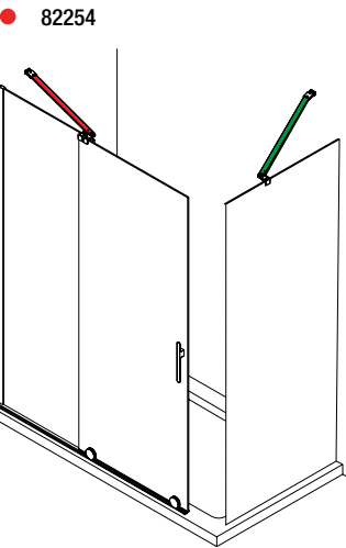
Mampara angular compuesta por un frontal, con tensor angular y con lateral fijo. (pag 164)
